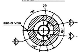
SECTION A-A SC 12
