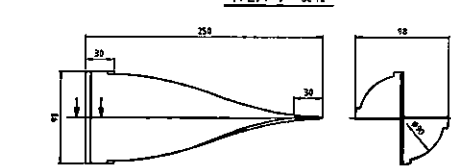
ITEM 7 SC 12
